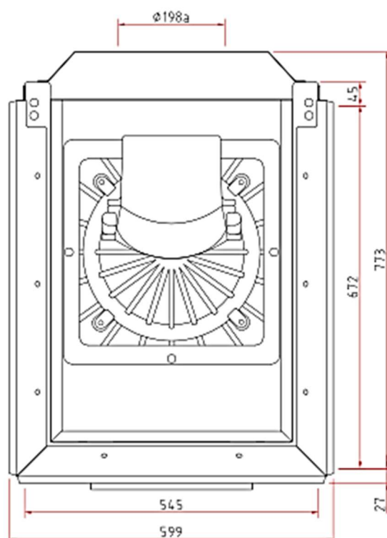
Draufsicht M 1:10
