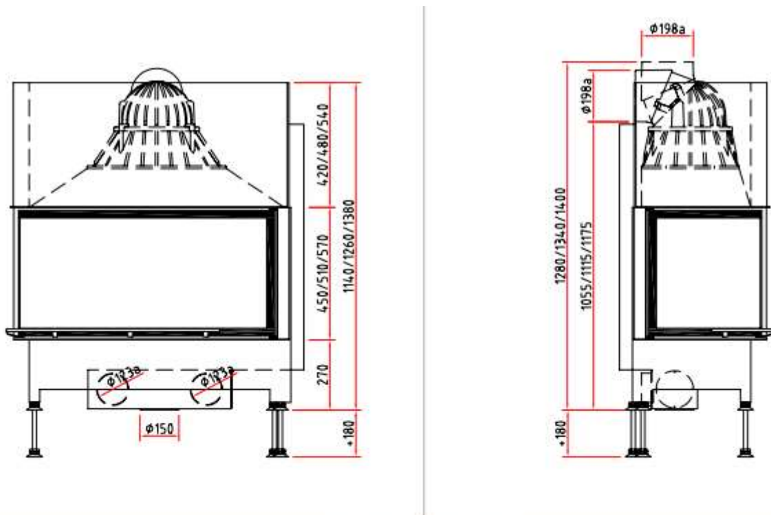
Draufsicht M 1:10
